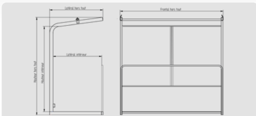
Garde-corps emboîtable
