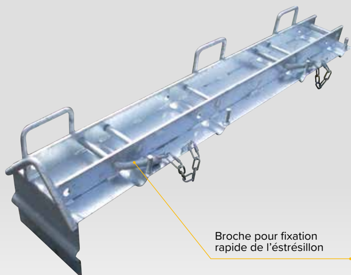
Barre de maintien du boisage
