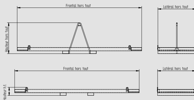
Option anse centrale avec élingue verrouillable
